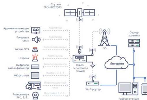
Рисунок 1 Схема подключения устройств
